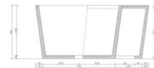
Widok cięcia 1-1
